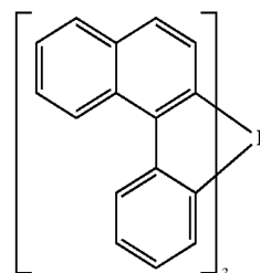
Ir(piq) 3
