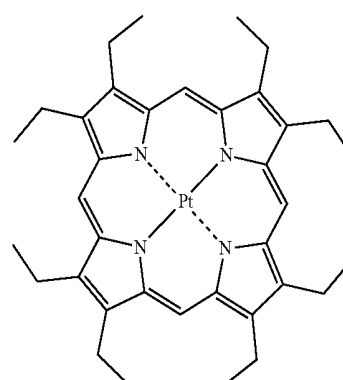
PtOEP
