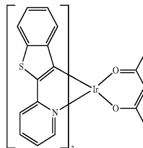
Btp 2 Ir(acac)
